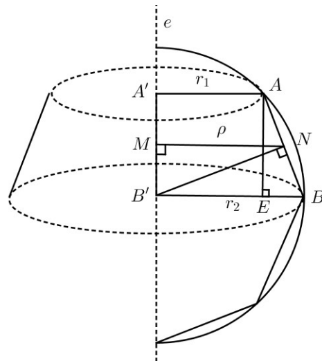
Figura 6: lateral de um tronco de cone gerada pela revolução do segmento.
