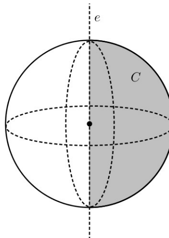
Figura 2: a esfera é um sólido de revolução.
