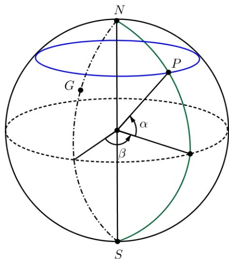
Figura 4: a latitude \alpha e a longitude \beta de um ponto P sobre a superfície da esfera.
