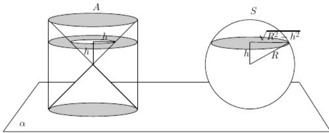
Figura 5: a esfera e a anti-clépsidra.
