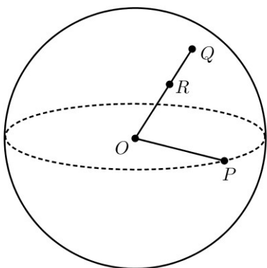
Figura 1: os pontos P e Q estão sobre a superfície esférica. O ponto R está na esfera correspondente.
