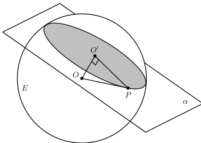
Figura 3: a interseção de uma esfera E e um plano \alpha .
