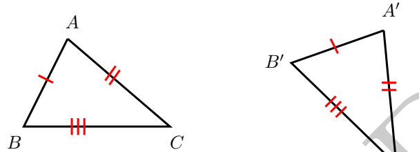
Figura 4: o caso de congruência LLL.
